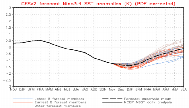
图 16 CFS.v2 预测
