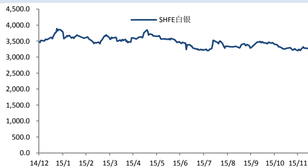
图4 沪银主力
