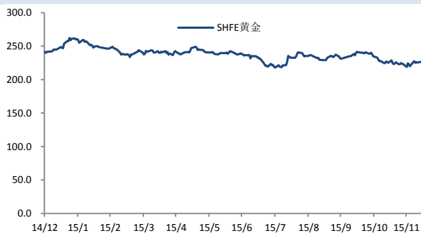
图3 沪金主力
